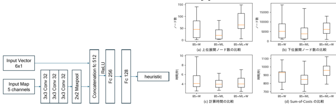
Fig. 1 左：提案モデル，右：シミュレーション結果 (BS：ビームサーチ，ML：機械学習，W：重み付き A*探索)
