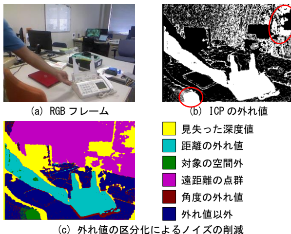
図1. 用いたRGBデータと位置合わせの結果得られたICPの外れ値。(a)動いている物体が写ったRGB画像。(b)対応するICPの外れ値。(c)外れ値の区分を表すカラーマップ。距離の外れ値(緑がかった青色)が提案手法で用いた外れ値。
